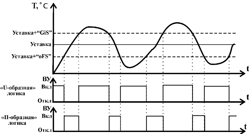
Рисунок 7: Пример работы ЛУ в режиме «I-образной» и «U-образной» логики.
